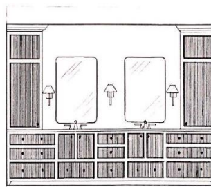
ELEVATION 2 - MASTER BATH SCALE: 3/4" = 1'-0"
